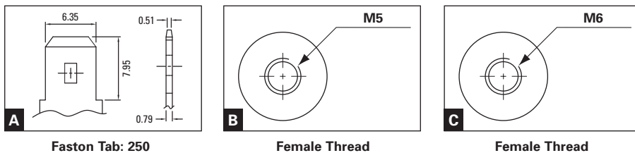
Faston Tab: 250
