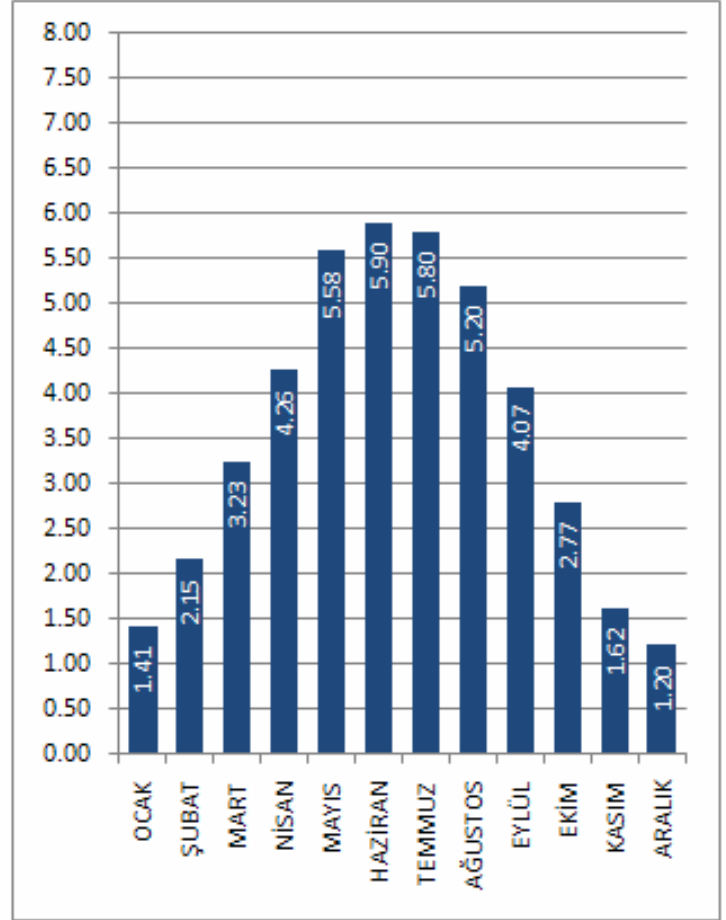
ZONGULDAK İLİ GLOBAL RADYASYON DEĞERLERİ (KWh/m 2 -gün)
