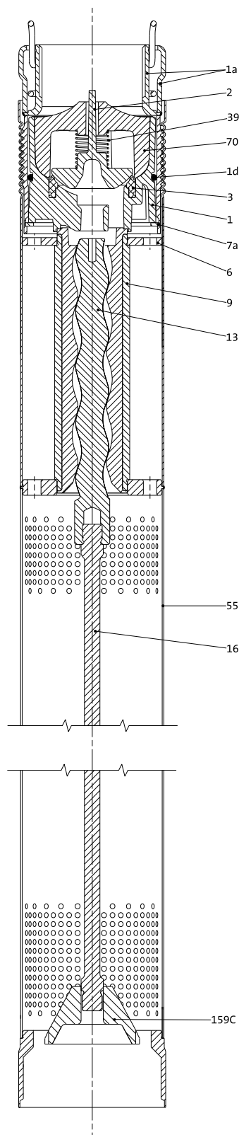
Fig. 29 Example: SQF 1.2-2
