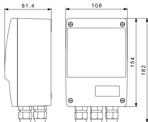
Fig. 22 Dimensions, CIU 273
