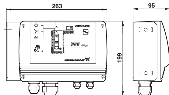
Fig. 19 Dimensions, CU 200
