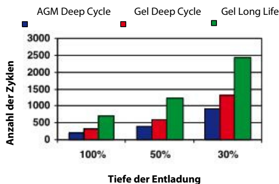
Bild 2: Zyklanzahl und Entladungstiefe
