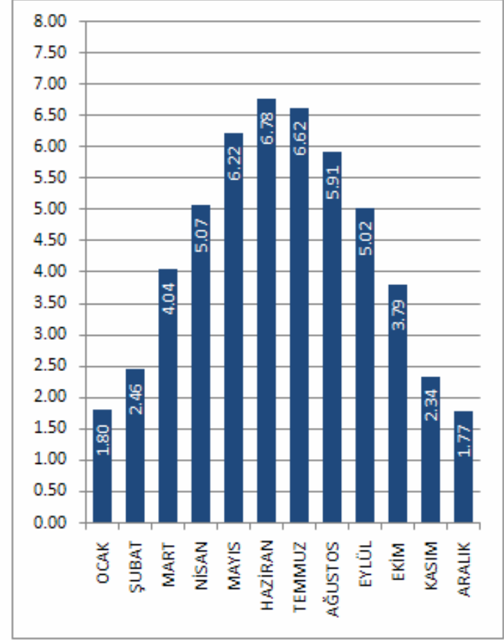
BATMAN İLİ GLOBAL RADYASYON DEĞERLERİ (KWh/m 2 -gün)
