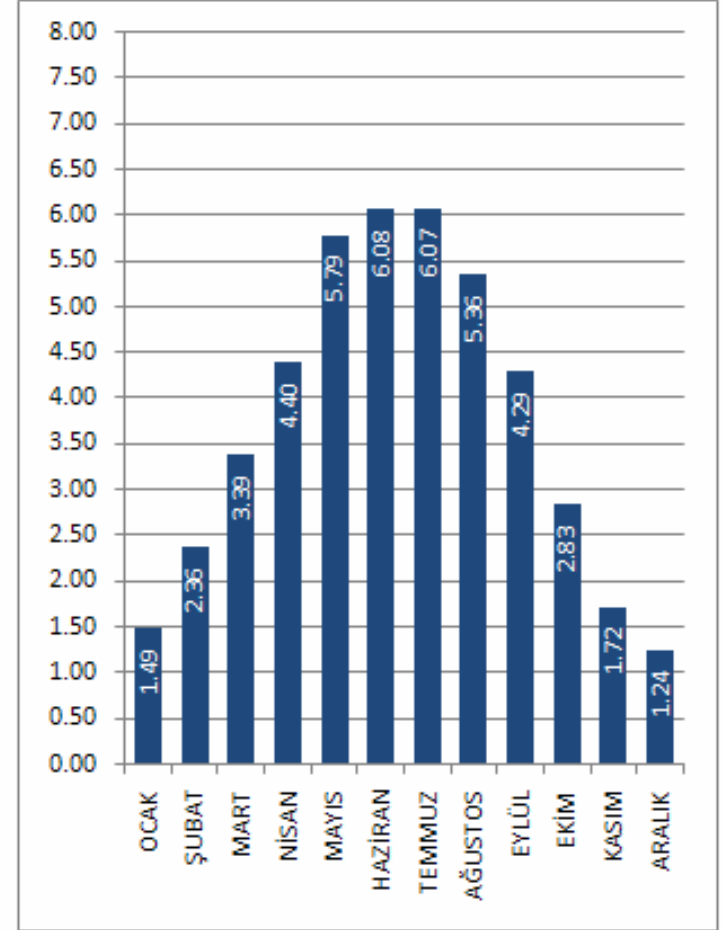
KARABÜK İLİ GLOBAL RADYASYON DEĞERLERİ (KWh/m 2 -gün)
