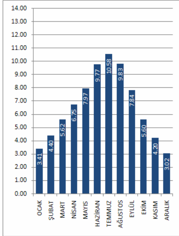
KARABÜK İLİ GÜNEŞLENME SÜRESİ DEĞERLERİ (Saat)
