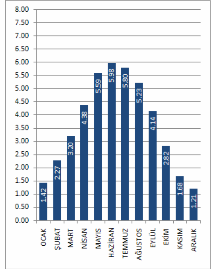
KOCAELİ İLİ GLOBAL RADYASYON DEĞERLERİ (KWh/m 2 -gün)
